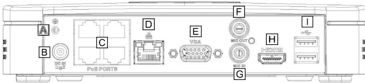
Abb. 1: Rückseite L-IPR-5104-P
